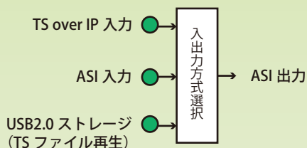
ブロック図 DBS7700
