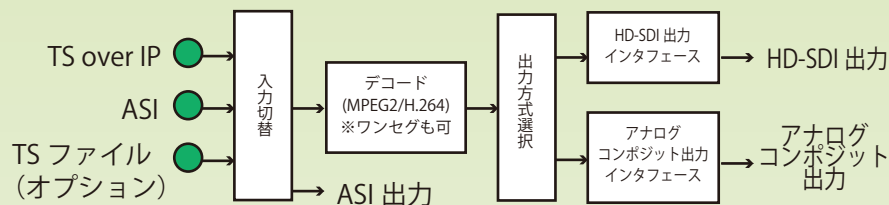
【ブロック図】
